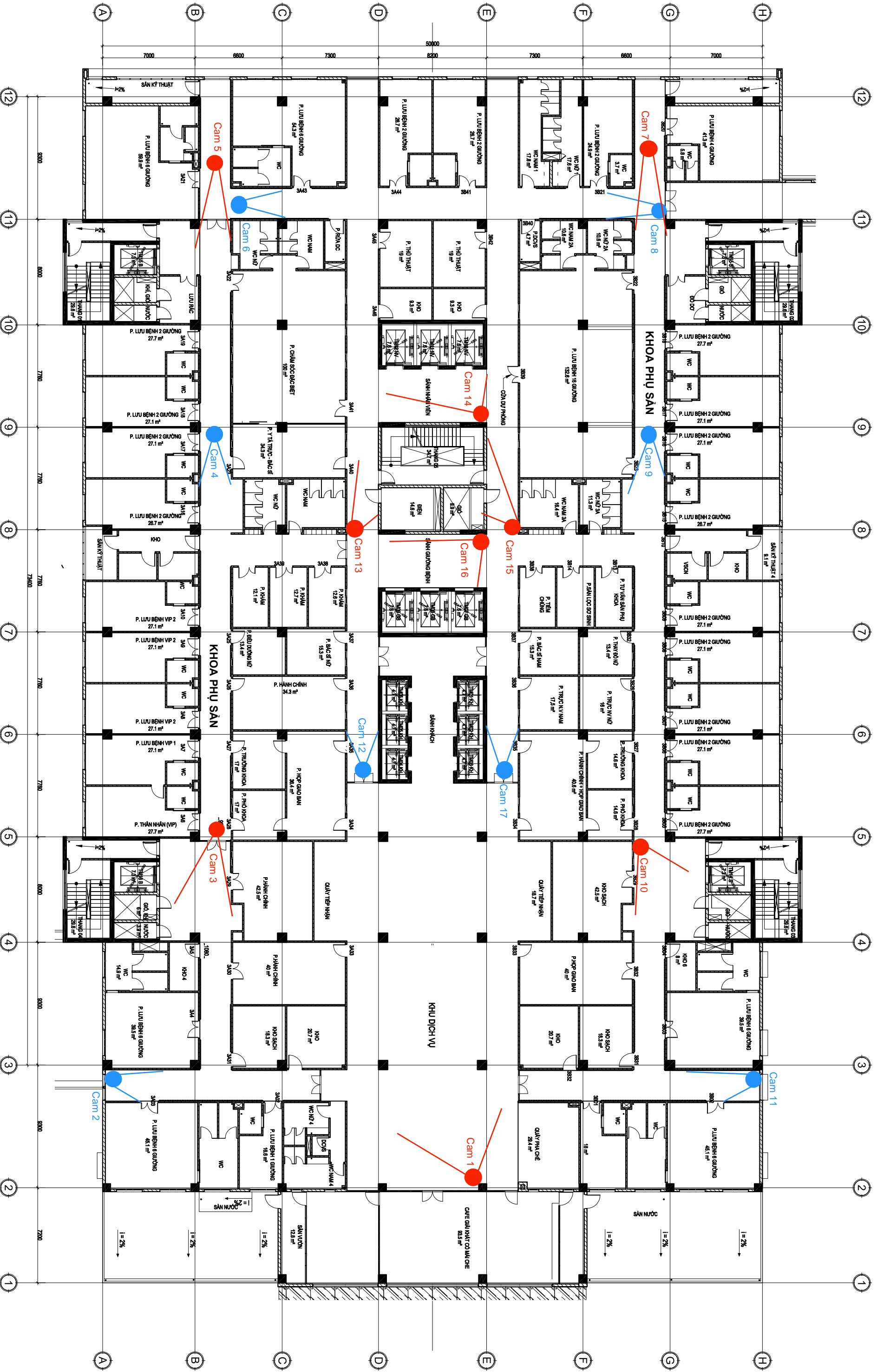
3 MẶT BẰNG CÔNG NĂNG TẦNG 3
